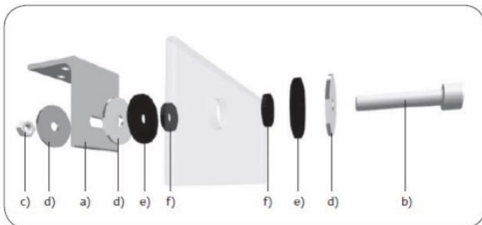
Abbildung 1: Befestigungskit
